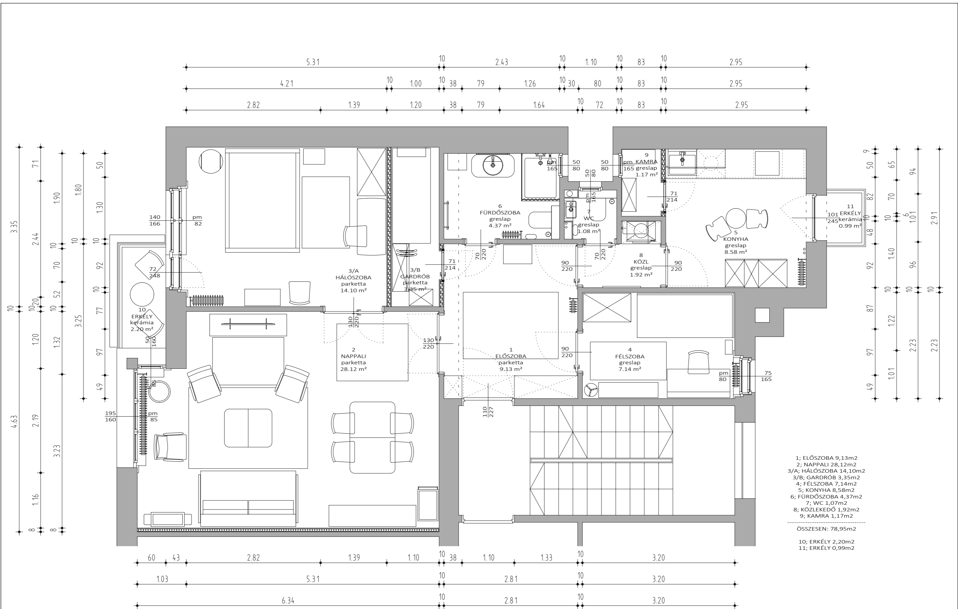
BERENDEZÉSI ALAPRAJZ 62360
